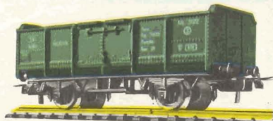
2009/SV Lit. 350 Carro scoperto a sponde alte a 2 assi tipo M della Società Veneta Ferrovie, nel suo tipico colore verde. Lunghezza fuori respingenti mm. 92
